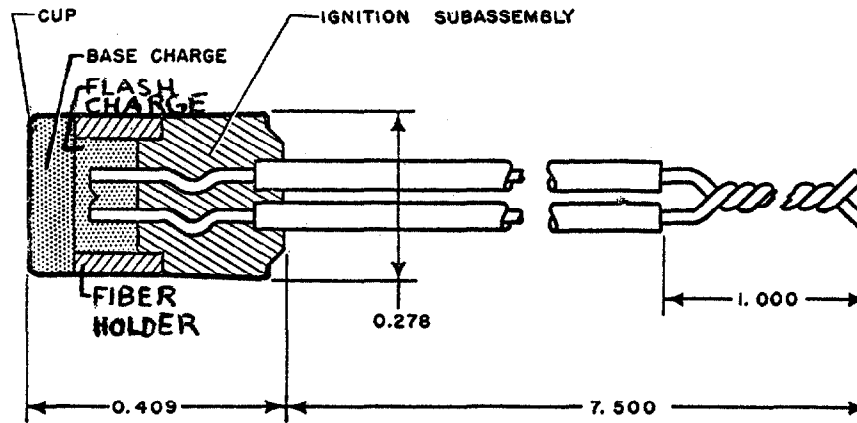
Fig 1-43 NAVY ELECTRIC FUZE PRIMER Mk112ModO
